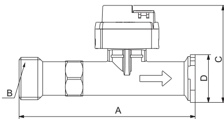
Рис. 74 Размеры, VFS QT, 2-40 л/мин, овальный фланец
